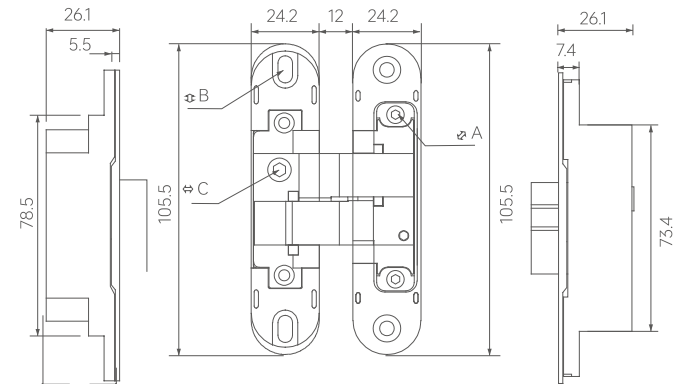
A: 前后调节 B: 上下调节 C: 左右调节
