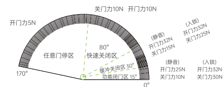
合页打开关闭力角度图（两只合页）
