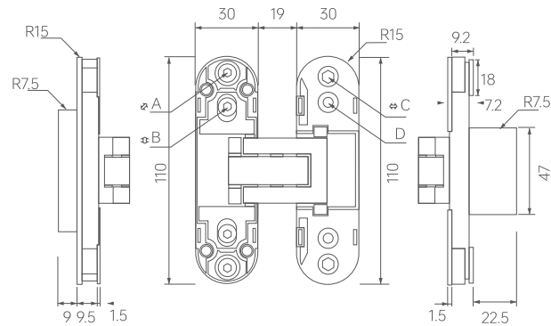
A: 前后调节 B: 上下调节 C: 左右调节
